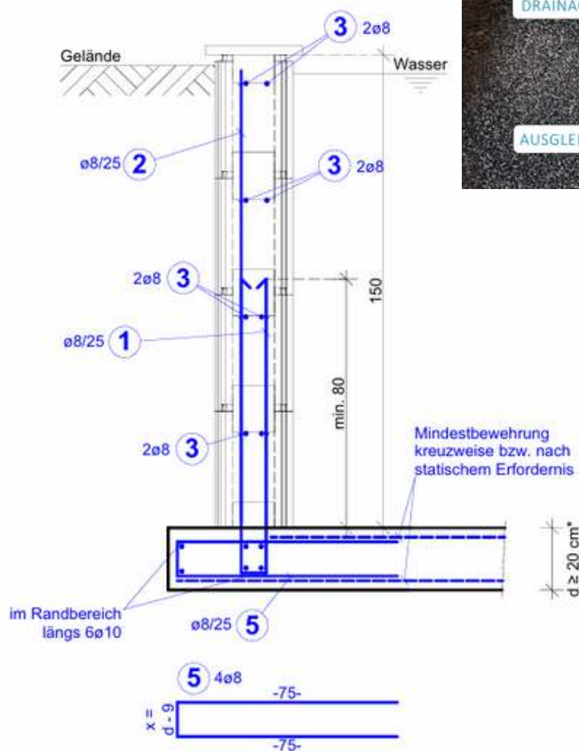
SCHNITT A - A M1:25
